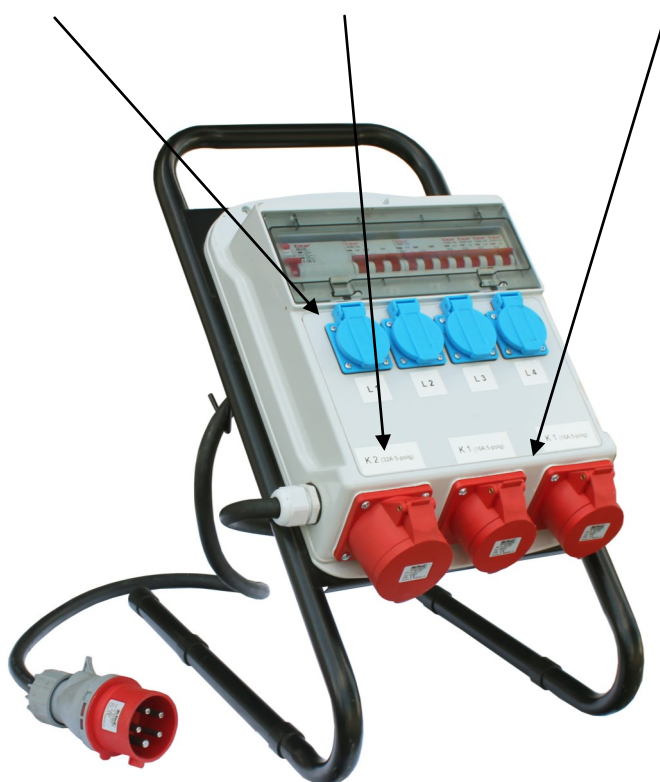
Afb. 1. De verdeelkast
